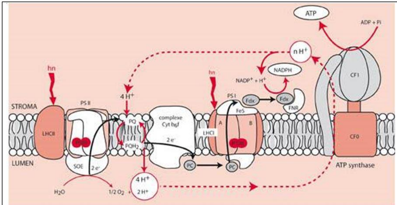
Figure 1 Schéma de transfert des électrons et protons dans les membranes des chloroplastes lors de la photosynthèse. PS1 (à droite) et PS2 (à gauche), complexe Cyt.B6f (entre les deux PS1 et PS2) et ATP synthase à droite de la figure. (Figure Morot-Gaudry et al. Dunod 2009.)
