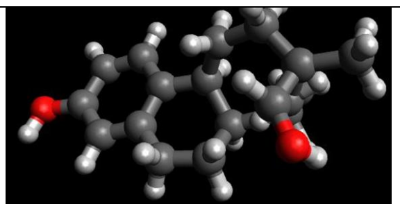
Figure 1 : molécule d'estradiol
