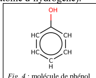
Fig. 4 : molécule de phénol
