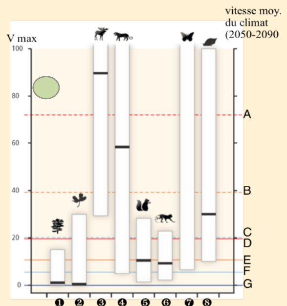
Figure 3. Vitesses maximum ( V_{max} ) auxquelles les espèces peuvent se déplacer dans des paysages (km/10 ans) d'après des observations et des modèles, comparées aux vitesses auxquelles les températures vont se déplacer selon les modèles prédictifs de changement climatique. Source : GIEC AR 5, 2014
