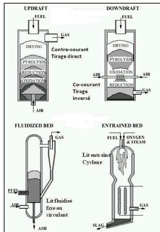
Figure 3. Types de réacteurs de gazéification : i) systèmes à lit fixe : gazéificateurs à co-courant (downdraft), et ceux à contre-courant (updraft) pour des installations mobiles, petites ou moyennes ; ii) systèmes à lit fluidisé, avec 3 catégories fonction de la vitesse de fluidisation, les lits fluidisés denses circulants et entraînés, pour des installations de grande taille.
